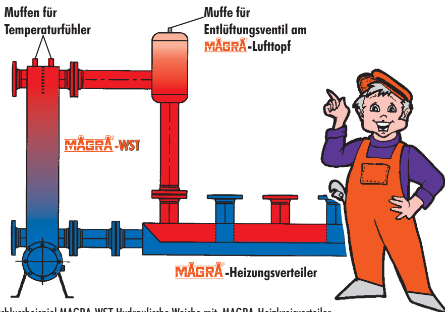
Anschlussbeispiel MAGRA-WST Hydraulische Weiche mit MAGRA-Heizkreisverteiler
